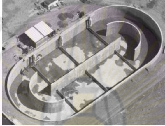
الشكل 7-12 صورة جوية لمحطة معالجة تعمل بطريقة خنادق الأكسدة.
