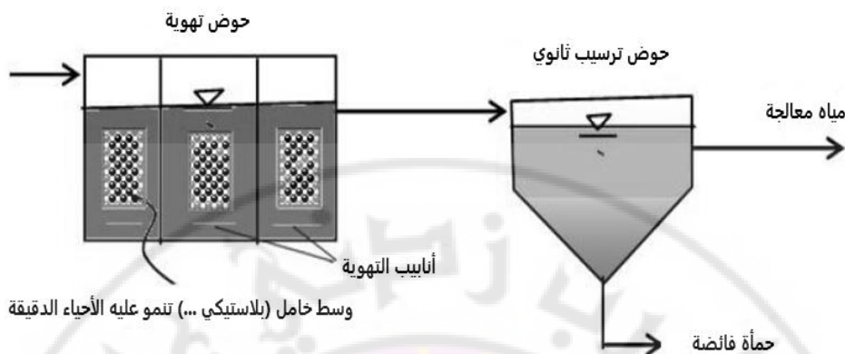
الشكل 8-12 طريقة النمو المتصل المغمور.
