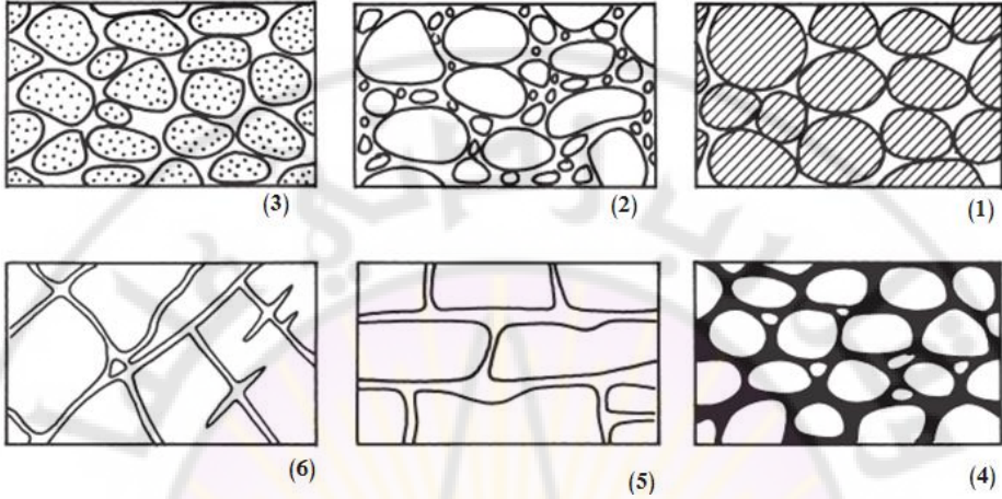
الشكل 8-1 أنماط المسامية مع علاقتها بالنسيج الصخري.
