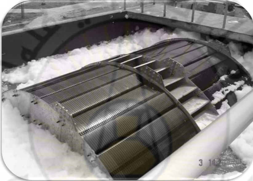
الشكل 5-12 الملامسات الحيوية الدورانية Rotating biological contactors RBCs.
