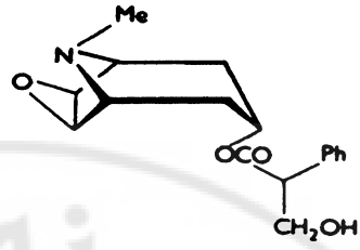
Hyoscine (Scopolamine)
