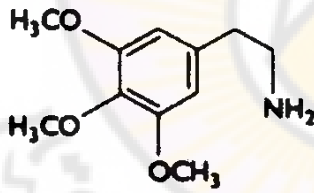
Mescaline
