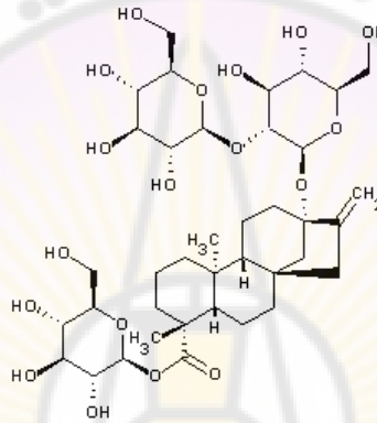
الشكل-215- الستيفوزيد
