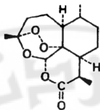
Artemisinin
