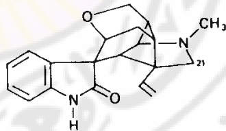
Gelsemine
