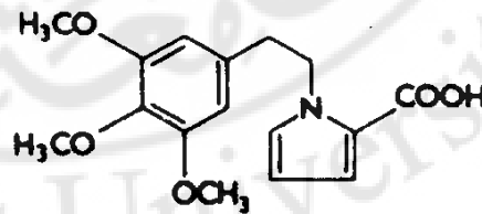
Peyonine
