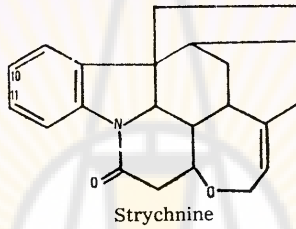
الشكل -168- الستركنين
