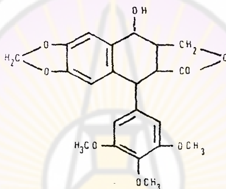
الشكل-192- البودوفيللوتوكسين
