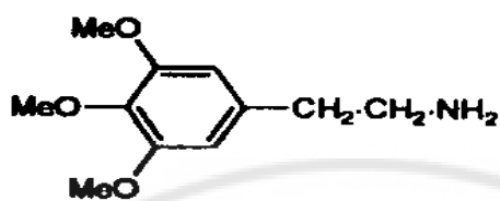
I, Mescaline
