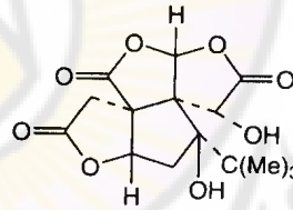
Bilobalide
