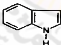
II,9 Indole
