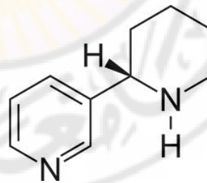
الشكل -114- الأنابازين
