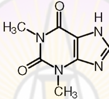
الشكل - 175- الثيوفيلين
