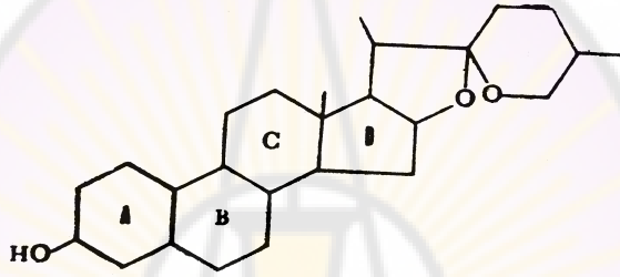
الشكل - Sarsapogenin-17
