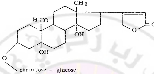
الشكل 55 - الكونفالوزيد
