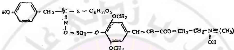
الشكل 97-السينالبين
