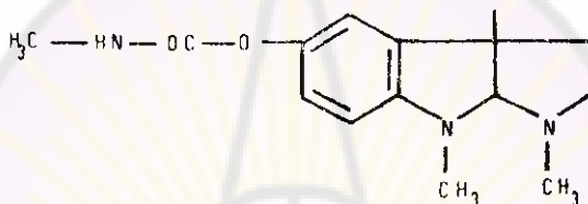
الشكل 166- الإيزرين
