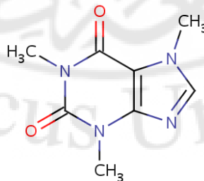
الشكل 173- الكافئين
