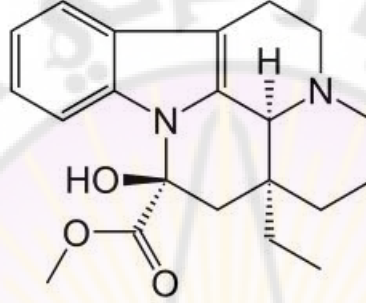
الشكل-164-قلويد الفينكامين
