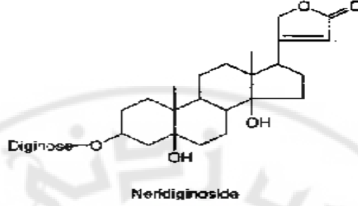
الشكل 50 - النيريديجينوزيد
