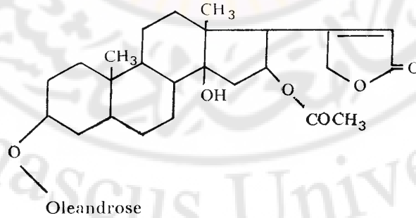
الشكل 51 - الأولياندرين
