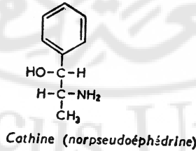
الشكل 136- القاتين
