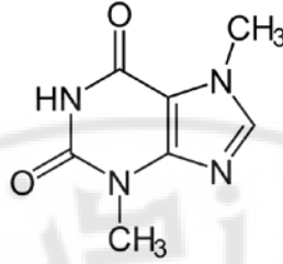
الشكل-174-التيوبرومين
