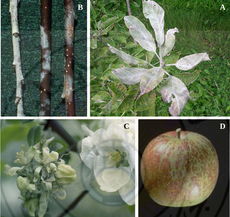
الشكل 3 - 11: أعراض الإصابة بمرض البياض الدقيقي على التفاح. (A) نموات حديثة مغطاة بنموات الفطر البيضاء الدقيقية المظهر. (B) أعراض الإصابة على الطرود الحديثة. (C) أعراض الإصابة على الأزهار. (D) قشرب على سطح الثمار نتيجة الإصابة.
