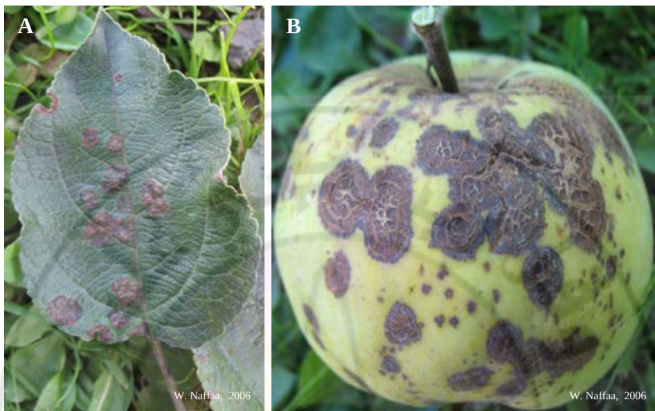
الشكل 3 – 65: أعراض الإصابة بجرب التفاح. A: أعراض الإصابة على الأوراق إذ يلاحظ وجود بقع دخانية اللون، ومجعدة على السطح العلوي للورقة. B: أعراض الإصابة على الثمار إذ تلاحظ البقع المتفلنة والمتشققة.
