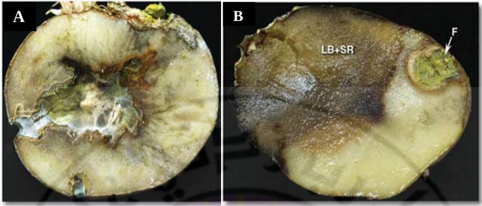
الشكل 3 - 52: A: تجويف داخل الدرنه مغطى بمشيجه الفطر. B: ظهور إصابة مشتركة بثلاثة أمراض على نفس الدرنه. ( LB+SR ) إصابة باللحة المتأخرة متبوعة بإصابة بالعفن الطري البكتيري. ( F ) إصابة بالعفن الجاف الفيوزاريومي.
