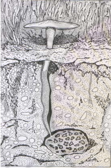
الشكل 2 - 3: ثمرة دعامية للفطر Termitomyces متشكلة على ساق شبه جذري Pseudorhiza نشأ من قرص للنمل الأبيض على مسافة 0.9 م تحت سطح التربة (عن TALBOT, 1971).
