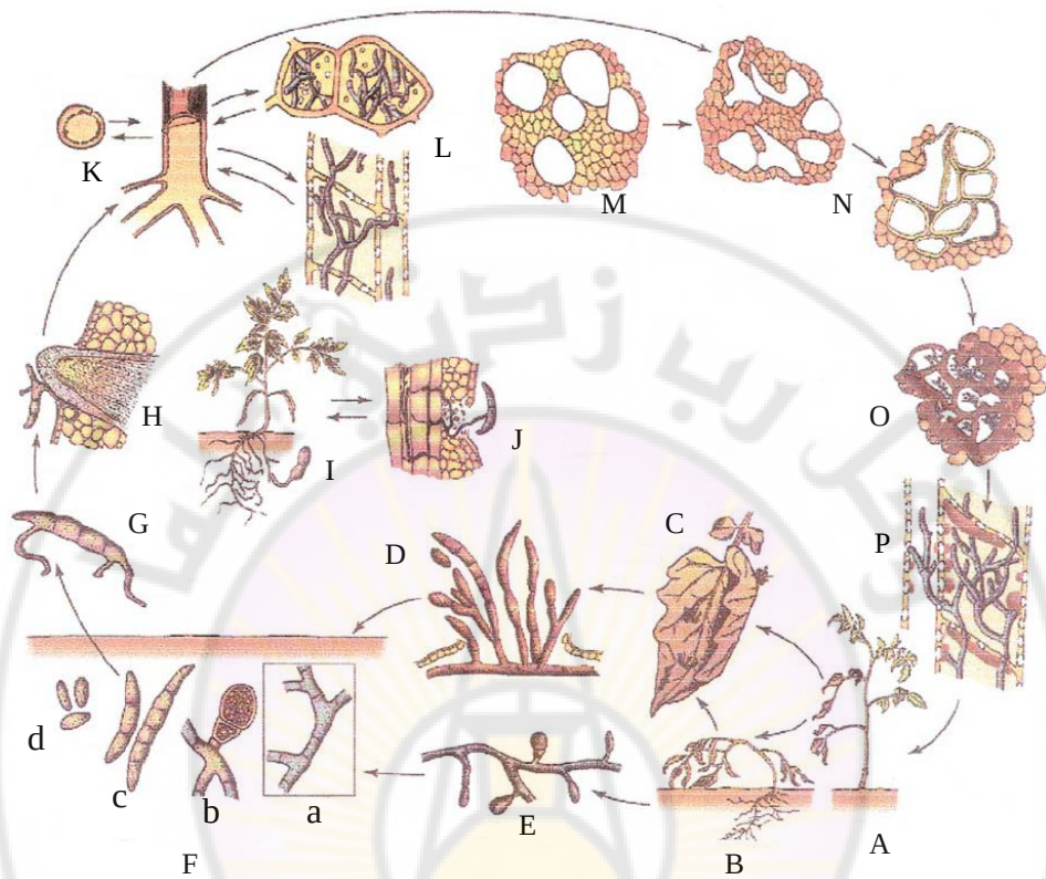
الشكل 3 – 74: دورة مرض ذبول البنندورة الفيوزاريومي المتسبب عن الفطر Fusarium oxysporum f. sp. lycopersici (عن Agrios, 2004).
