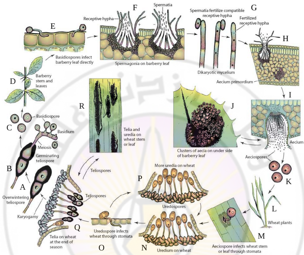
الشكل 3 - 27: دورة مرض صدأ الساق على القمح (عن Agrios, 2004)
