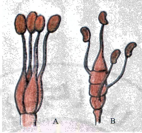
الشكل 2 – 22: أشكال مختلفة من الدعامات المقسمة طولياً أو عرضياً (A) الفطر Phragmobasidia . (B) الفطر Tremella . Auricularia .
