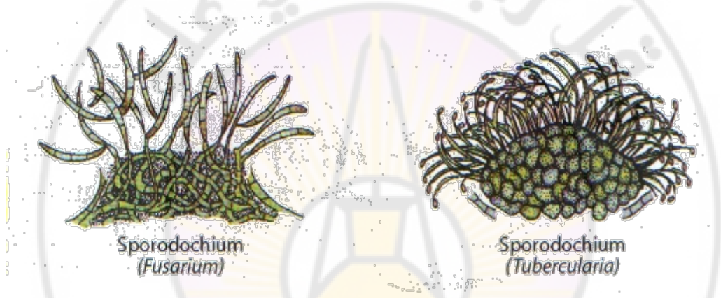
الشكل 2 - 26: مخطط تمثيلي للـ Sporodochium.
