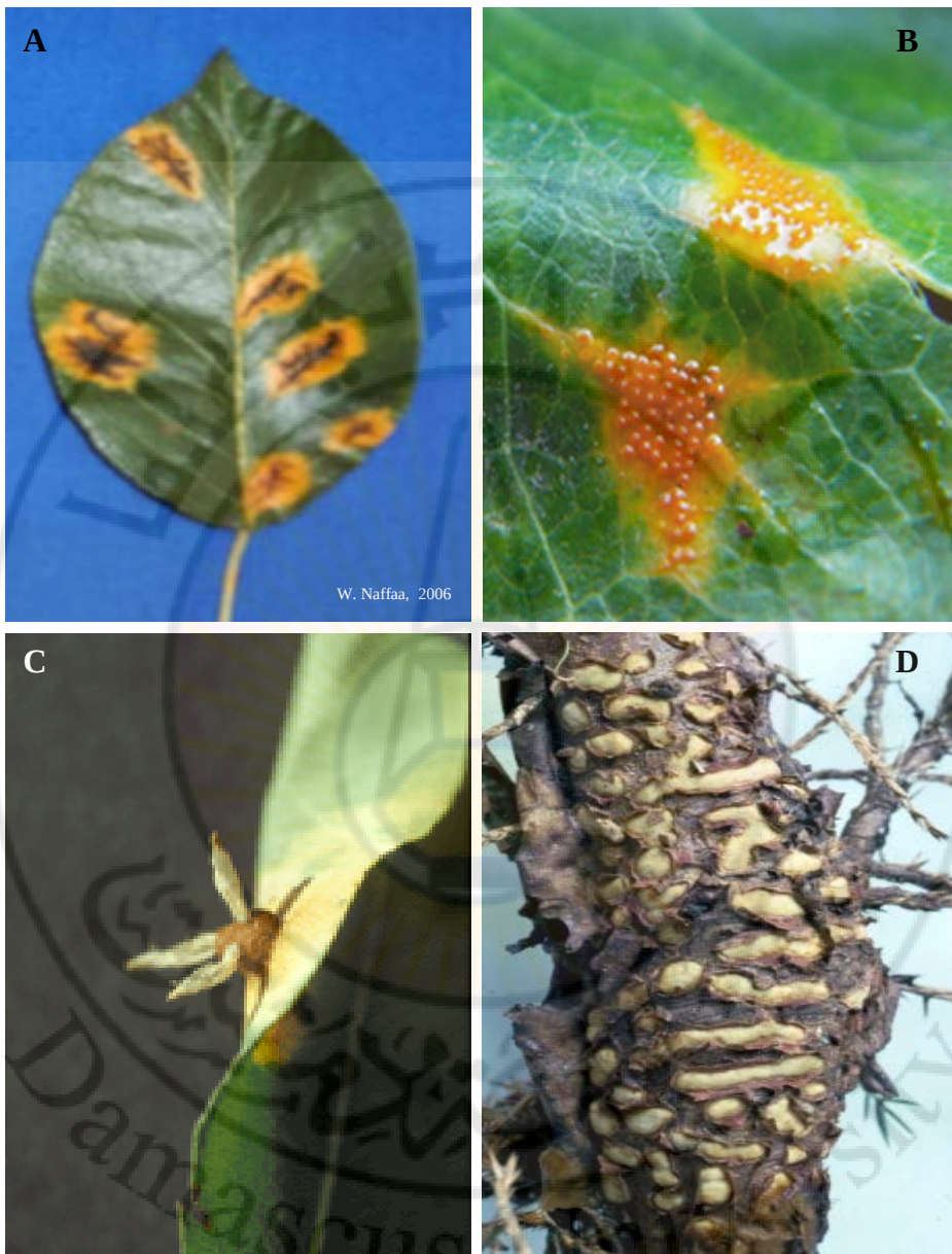
الشكل 3 – 33: أعراض الإصابة بمرض صدأ الكمثرى المتسبب عن الفطر Gymnosporangium sabinae . (A) بقع برتقالية على السطح العلوي لورقة الكمثرى، وتلاحظ الأوعية السبرموغونية في الوسط. (B) صورة مكبرة للأوعية السبرموغونية برتقالية اللون. (C) تدرن على السطح السفلي للورقة، وتخرج الأوعية الأسيدية مغزلية الشكل من محيطه. (D) انتفاخ أو تورم على أفرع العرعر.
