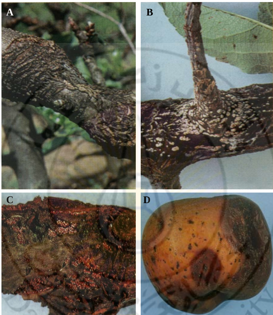
الشكل 3 - 107: أعراض الإصابة بمرض التقرح النكتيري على التفاح المتسبب عن الفطر Nectria galligena . (A) تأكل منطقة التقرح وظهور الخشب الميت تحت المنطقة المتقرحة. (B) مطارح الفطر الكونيدية المتشكلة على منطقة تقرح حديثة. (C) ثمار زرقية حمراء اللون متشكلة على منطقة تقرح قديمة. (D) أعفان متشكلة على الثمار خلال فترة التخزين (عن Giraud et al., 1996).
