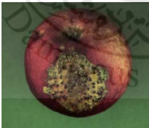
الشكل 3 – 30: أعراض الإصابة بالفطر Gymnosporangium juniperi-virginiana على ثمار التفاح إذ تلاحظ الأوعية السبرموغونية في وسط البقعة و الأوعية الأسيدية في المحيط.
