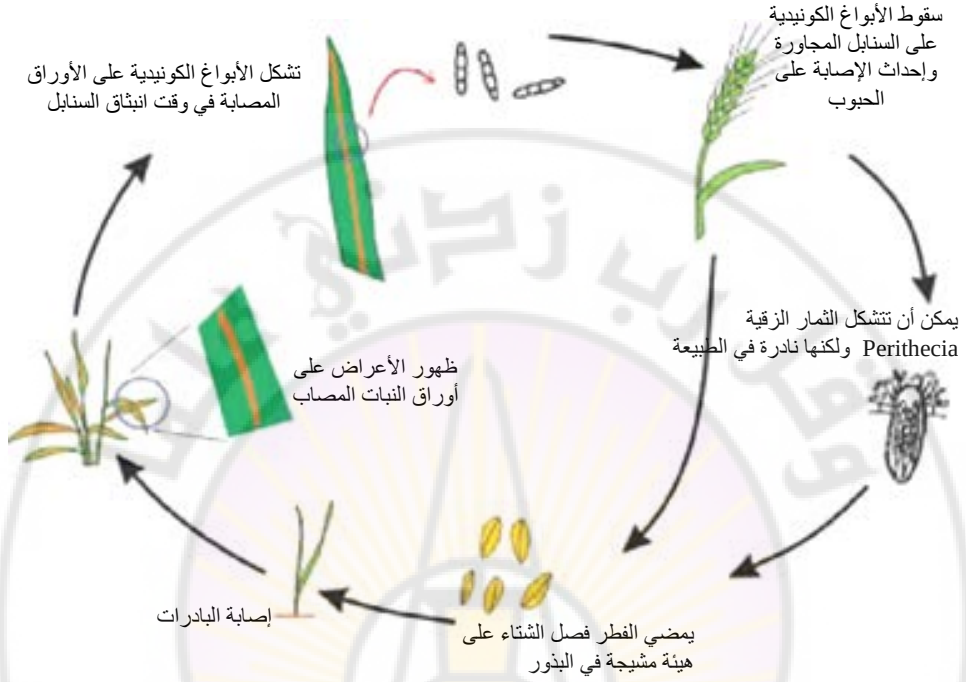
الشكل 3 - 95 : دورة مرض التخطط المتوازي على الشعير المتسبب عن الفطر Pyrenophora graminea .
