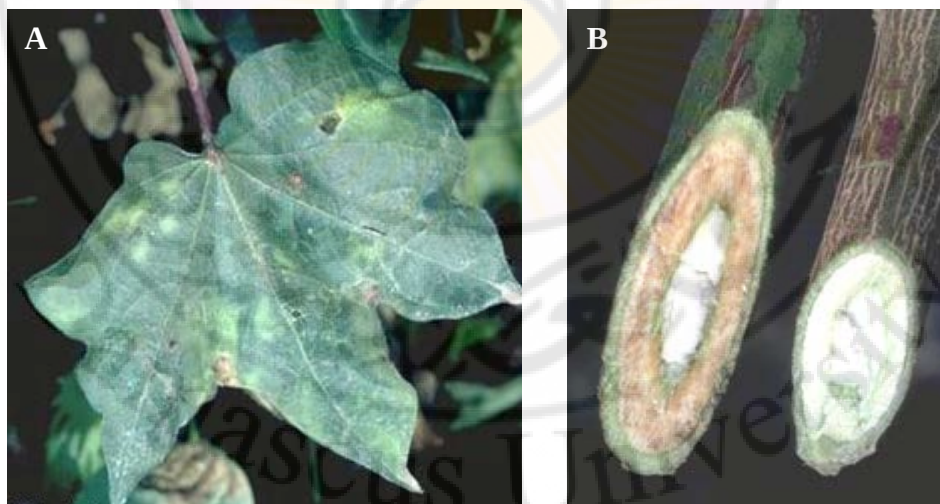
الشكل 3 – 75: أعراض الإصابة بالذبول الفريسيومي على القطن المتسبب عن الفطر Verticillium dahliae . A: بقع شاحبة على حافة الورقة وبين العروق. B: مقطع عرضي يبين تلون الأوعية الناقلة في ساق نبات مصاب بالذبول مقارنة مع لون الأوعية الناقلة في ساق نبات سليم.
