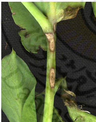
الشكل 3 - 87: أعراض الإصابة بلفة الأسكوكيتا على البازلاء. إذ يلاحظ على حواف الأوراق ظهور لطح غير منتظمة الشكل بلون بني داكن أو مسود. كما يلاحظ على الساق ظهور بقع بيضوية الشكل.
