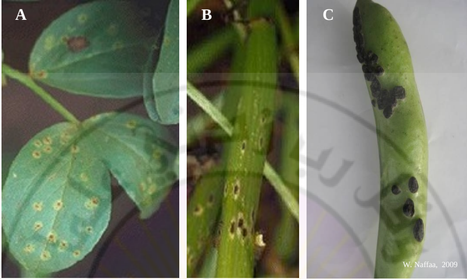
الشكل 3 – 38: أعراض الإصابة بصدأ الفول. A: البثرات اليوريدية على السطح العلوي لوربقات الفول. B: بثرات تيلييتية بيضاوية الشكل على الساق. C: بثرات تيلييتية دائرية الشكل وسوداء اللون على قرون الفول.
