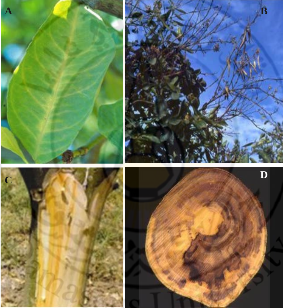
الشكل 3 – 118: أعراض الإصابة بمرض مالنيسكو على الحمضيات. (A) اصفرار عروق الأوراق. (B) موت تراجعي للأفرع متركزة على جهة واحدة من الشجرة. (C) تلون الخشب باللون البرتقالي في الأشجار المصابة. (D) تلون قلب الخشب باللون البني نتيجة الإصابة المزمنة بالمرض "Mal nero".
