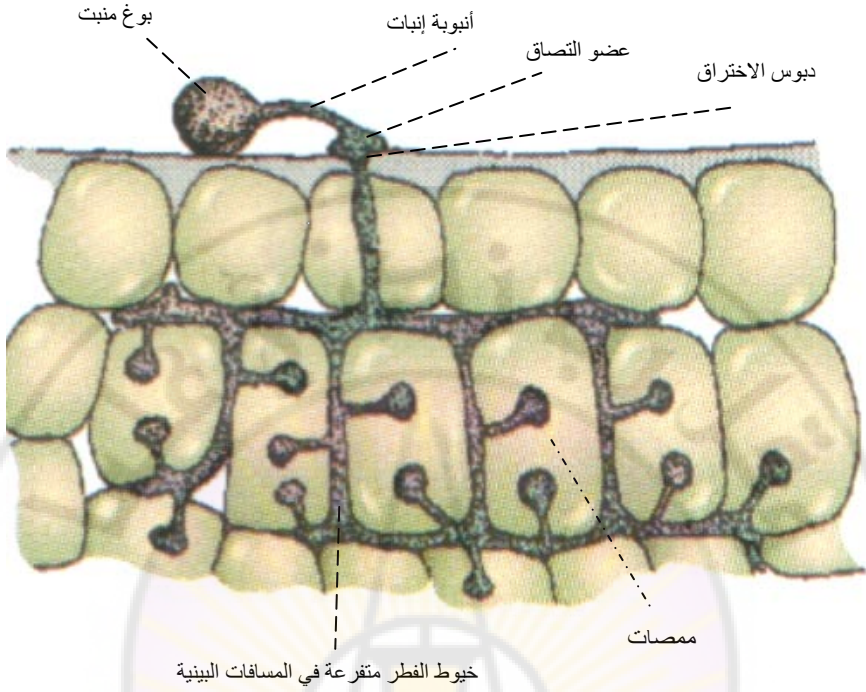
الشكل 2 - 8: أعضاء الالتصاق Appressoria التي تتشكل عند ملاصقة أنبوبة الإنبات لسطح الورقة.
