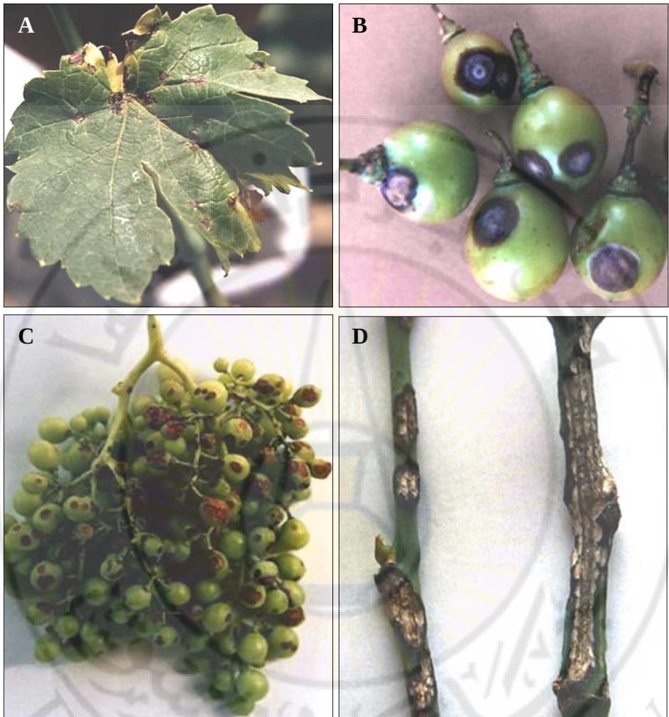
الشكل 3 - 105: أعراض الإصابة بمرض أنثراكنوز الكرمة. (A) بقع بنية داكنة أو مسودة على الأوراق، مركزها رمادي ومحيطها داكن. (B) أعراض الإصابة على الثمار بشكل بقع دائرية، مركزها رمادي، ومحاطة بإطار أسود - بنفسجي. (C) العديد من البقع البنية الداكنة، والغائرة قليلاً على سطح الحبات. (D) لطخ متطاولة، ومتفرحة على الطرود، رمادية اللون في المركز، ومحاطة بنسيج إلتحامي داكن اللون، ومرتفع قليلاً عن السطح.
