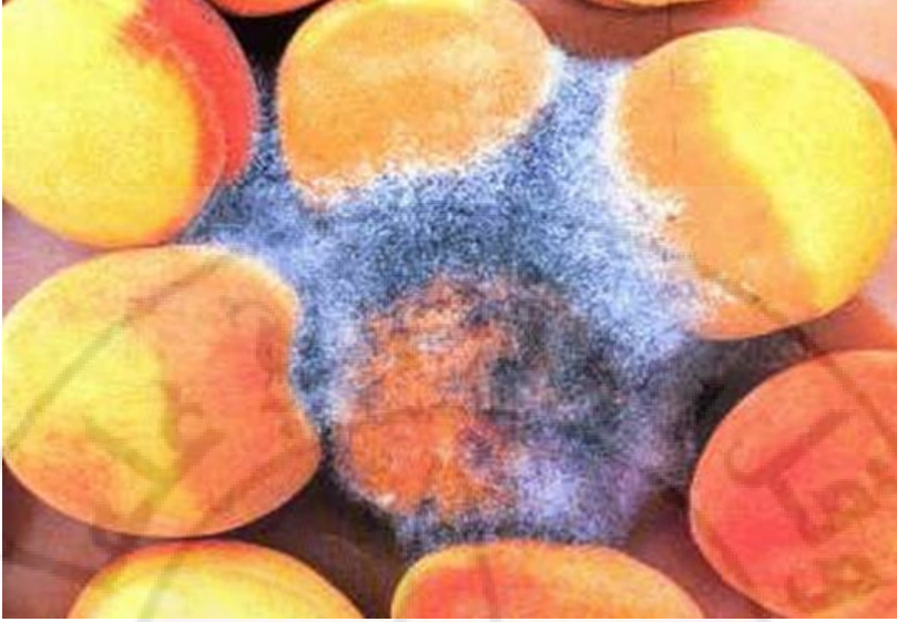
الشكل 3 – 61: أعراض الإصابة بالعفن الطري على الدراق. إذ تلاحظ نموات الفطر السوداء الرمادية نتيجة تشكل الأكياس البوغية السبورانجية.
