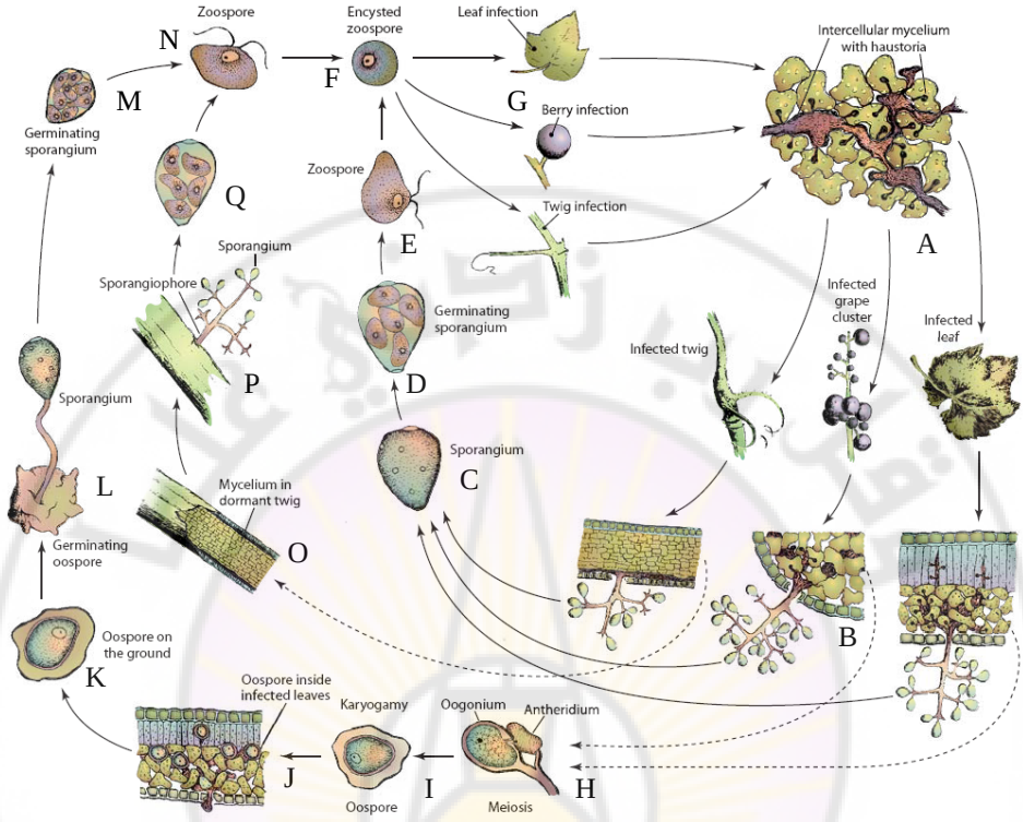
الشكل 3-3 : دورة حياة الفطر Plasmopara viticola (عن Agrios, 2004)
