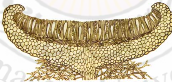
الشكل 2 - 19 : مقطع عرضي في ثمرة زقية من الطراز الطبقي Apothecium
