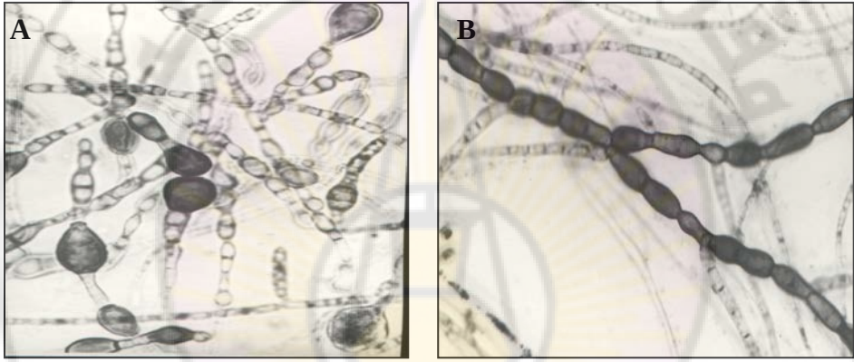
الشكل 2 - 11: (A) أبواغ كلاميدية طرفية وبيئية. (B) تحول كل خلايا المشيجة إلى أبواغ مقاومة تدعى بالمشيجة الساكنة Resting mycelium. (عن فضول)
