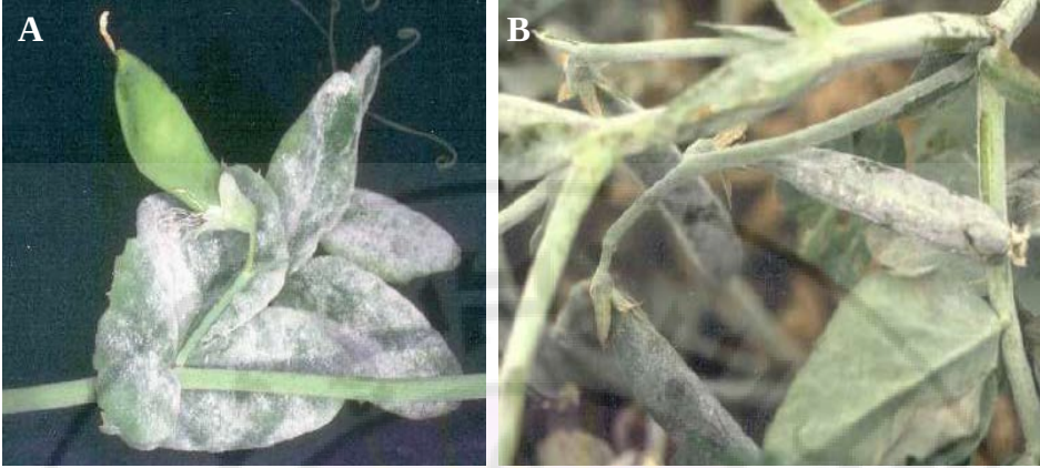
الشكل 3 - 14: أعراض الإصابة بالبياض الدقيقي على البازلاء. (A) طبقة دقيقية بيضاء تغطي الأوراق. (B) قرون مغطاة بشكل كامل بنموات الفطر الرمادية أو المائلة إلى الزرقاء.
