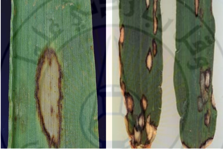
الشكل 3 - 97 : أعراض الإصابة بمرض السفعة الحقلية على الشعير المتسبب عن الفطر Rhynchosporium secalis إذ تلاحظ على أنصال الأوراق بقع بيضوية أو مستطيلة مبيضة أو قشبية اللون في المركز وذات حواف بنية داكنة.
