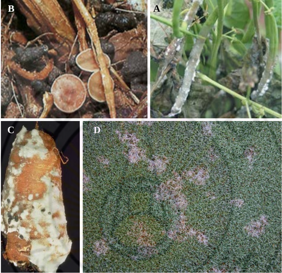
الشكل 3 – 56: أعراض الإصابة بأمراض السكليروتينيا. (A) مشيجة قطنية بيضاء على قرون الفاصولياء. (B) أجسام حجرية سوداء اللون، وقد أنبت البعوض منها إلى ثمار زقية قرصية. (C) عفن أبيض على الجزر مع ملاحظة وجود بعض الأجسام الحجرية سوداء اللون. (D) أعراض الإصابة بمرض بقعة الدولار على نباتات المروج.
