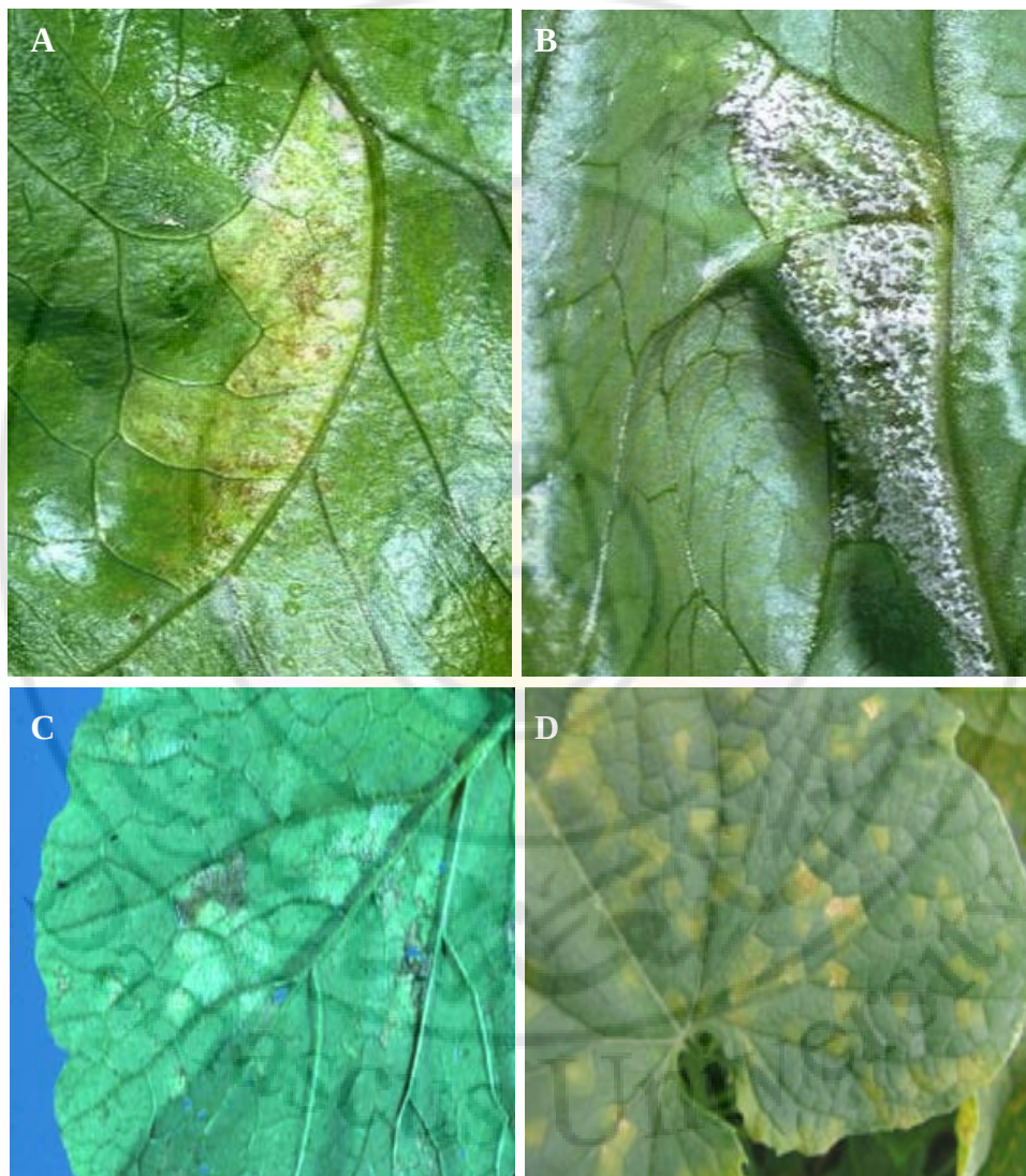
الشكل 3 - 6: أعراض الإصابة بالبيضاء الزغبية. (A) بقع صفراء شاحبة على السطح العلوي لأوراق الخس. (B) زغب أبيض على السطح السفلي لأوراق الخس. (C) أعراض الإصابة على الصليبيات. (D) أعراض الإصابة على القرعيات.
