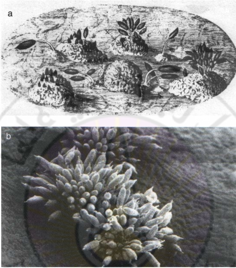
الشكل 1 - 1: مظهر لنفس التراكيب الفطرية (البثرات) على ورقة ورد مصابة بمرض الصدأ المتسبب عن الفطر Phragmidium rosae (بفاصل زمني يزيد عن 300 سنة). (a) رسم تخطيطي حسب Hook عام 1665. (b) صورة مأخوذة بالمجهر الإلكتروني في عام 1987. (عن Lepoivre, 2003).
