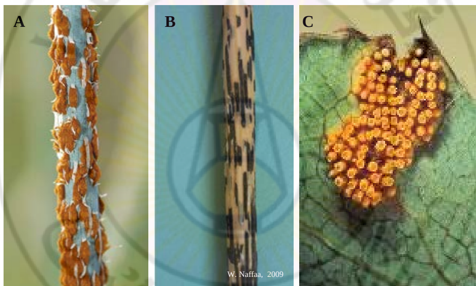
الشكل 3 – 26: أعراض الإصابة بمرض صدأ الساق على القمح. (A) بثرات يوريدية برتقالية اللون على الساق. (B) بثرات تيليتية سوداء اللون ومتحدة على شكل أشرطة طويلة. (C) أوعية أسيدية على السطح السفلي لورقة نبات البربريس.
