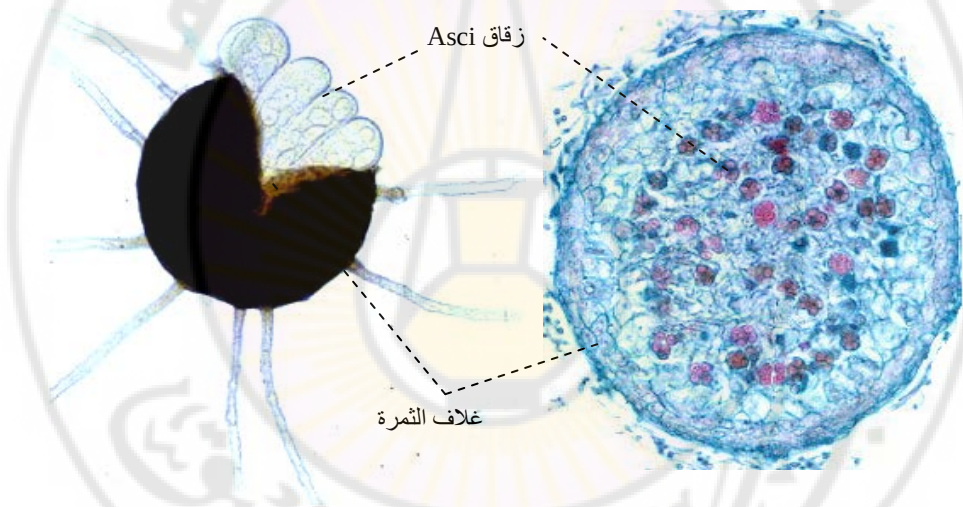
الشكل 2 - 17: ثمرة زقية مغلفة Cleistothecium. (A) ثمرة زقية لفطريات البياض الدقيقي. (B) مقطع في ثمرة زقية مغلفة إذ يلاحظ توزع الزقاق بداخلها بدون انتظام .
