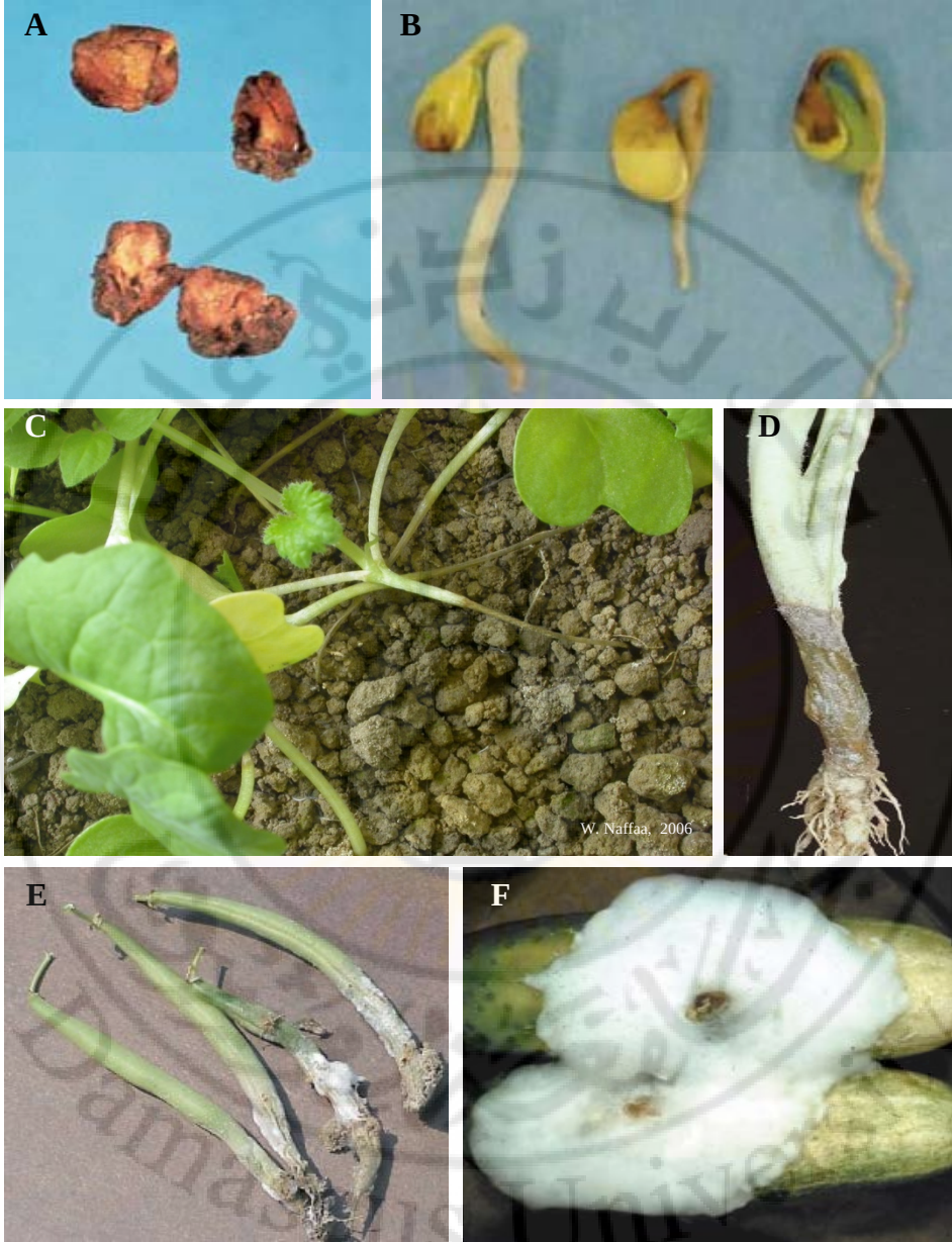
الشكل 3 - 58: (A) تحلل البذار. (B) إصابة بادرات الفول قبل خروجها فوق سطح التربة. (C) سقوط بادرات اللفت الزيتي بعد خروجها فوق سطح التربة. (D) إصابة قاعدة ساق التبنغ. (E) عفن طري على قرون الفاصولياء الخضراء، و (F) على الخيار، إذ تلاحظ نموات الفطر القطنية على الأنسجة المصابة.
