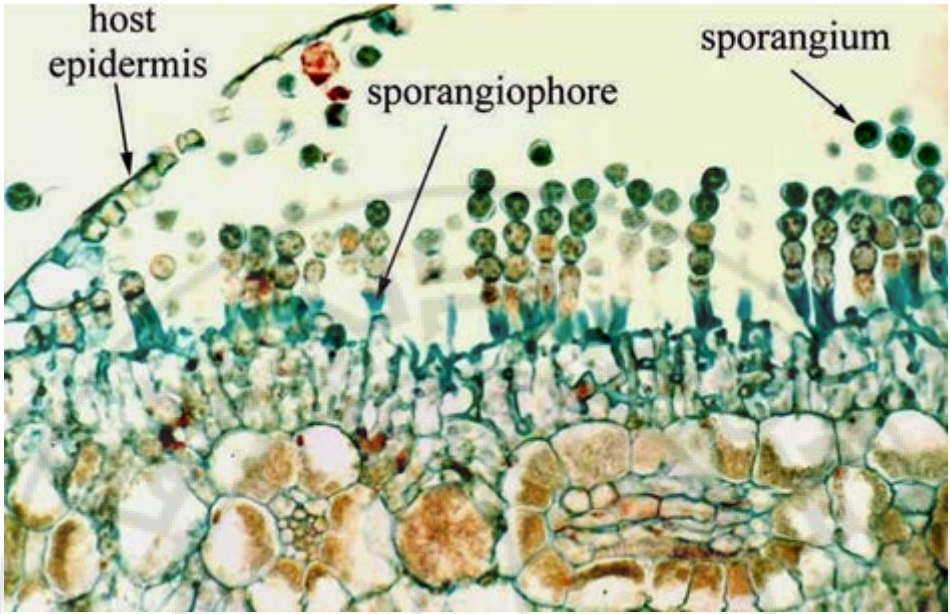
الشكل 3 - 114: بثرة للفطر Albugo candida المسبب لمرض الصدأ الأبيض على الصليبيات، إذ يلاحظ تمزق بشرة النبات تحت ضغط الأبواغ عليها. كما يلاحظ تشكل الأبواغ في سلاسل على حوامل قصيرة صولجانية الشكل.
