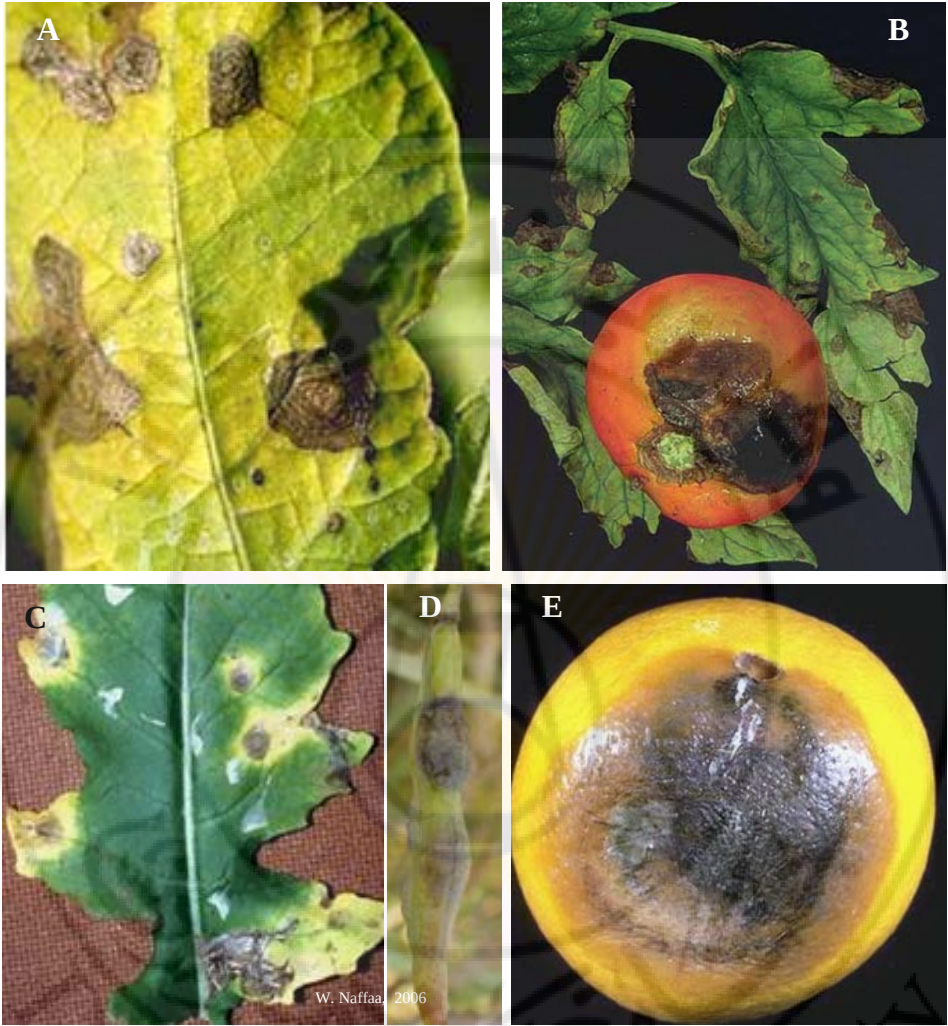
الشكل 3 – 90: أعراض الإصابة ببعض أمراض الألترناريا. (A) تبقعات على شكل حلقات متداخلة على أوراق البطاطا مصابة بمرض اللفة المبكرة المتسبب عن الفطر Alternaria solani . (B) تبقعات على أوراق وثمار البندورة مصابة أيضاً بمرض اللفة المبكرة. (C) تبقعات سوداء على أوراق نبات اللفت الزيتي، و (D) على القرون، ناتجة عن الإصابة بالفطر A. brassicae . (E) أعراض الإصابة على ثمار الحمضيات.
