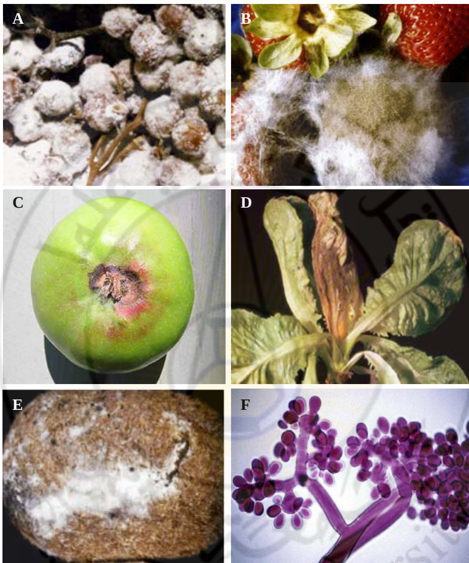
الشكل 3 – 53: أعراض الإصابة بالفطر Botrytis cinerea . A: عفن رمادي على عناقيد العنب. B: عفن رمادي على ثمار الفريز. C: عفن الطرف الزهري على ثمار التفاح. D: عفن رمادي على الخس. E: عفن رمادي على ثمار الكيوي. F: حوامل وأبواغ كونيدية للفطر Botrytis sp. إذ يلاحظ أن الخلية القمية في تفرعات الحامل البوغي مستديرة وتحمل مجموعات من الأبواغ الكونيدية على شكل عناقيد العنب.
