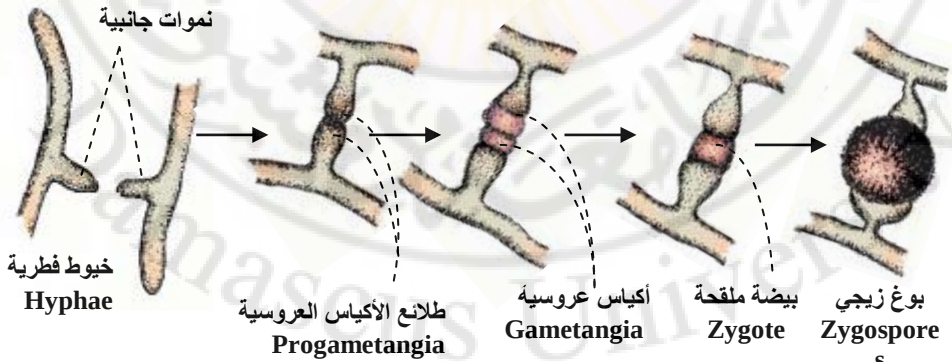
الشكل 2 – 14: مراحل تشكل البوغ الزيجي Zygospore عند الفطريات الزيجية.
